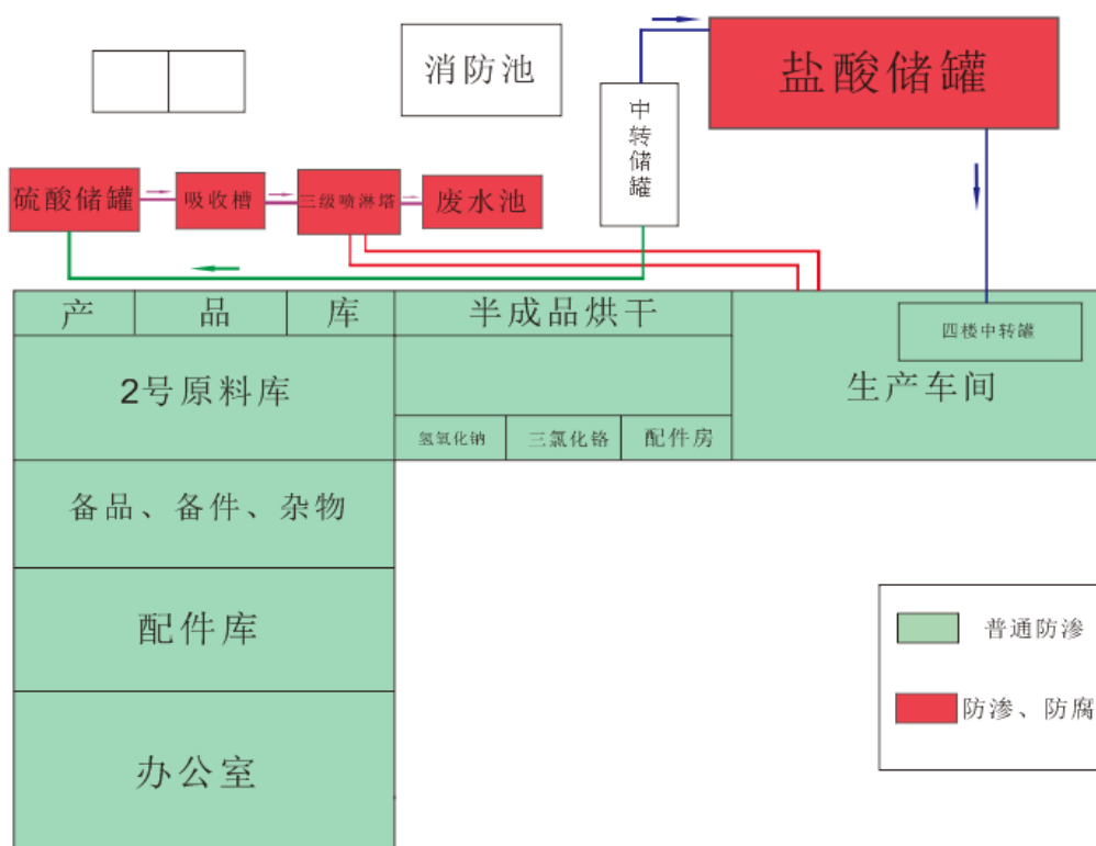
图 3-3 厂区管网图
