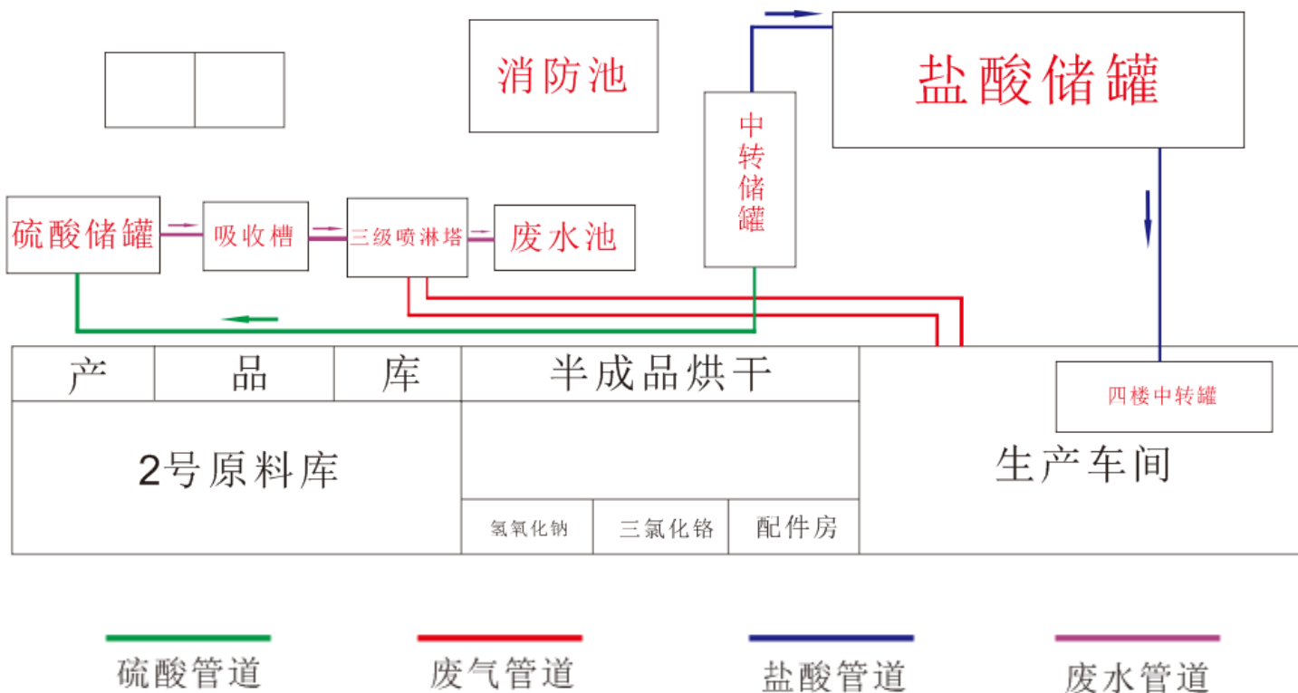
图 3-3 厂区管网图
